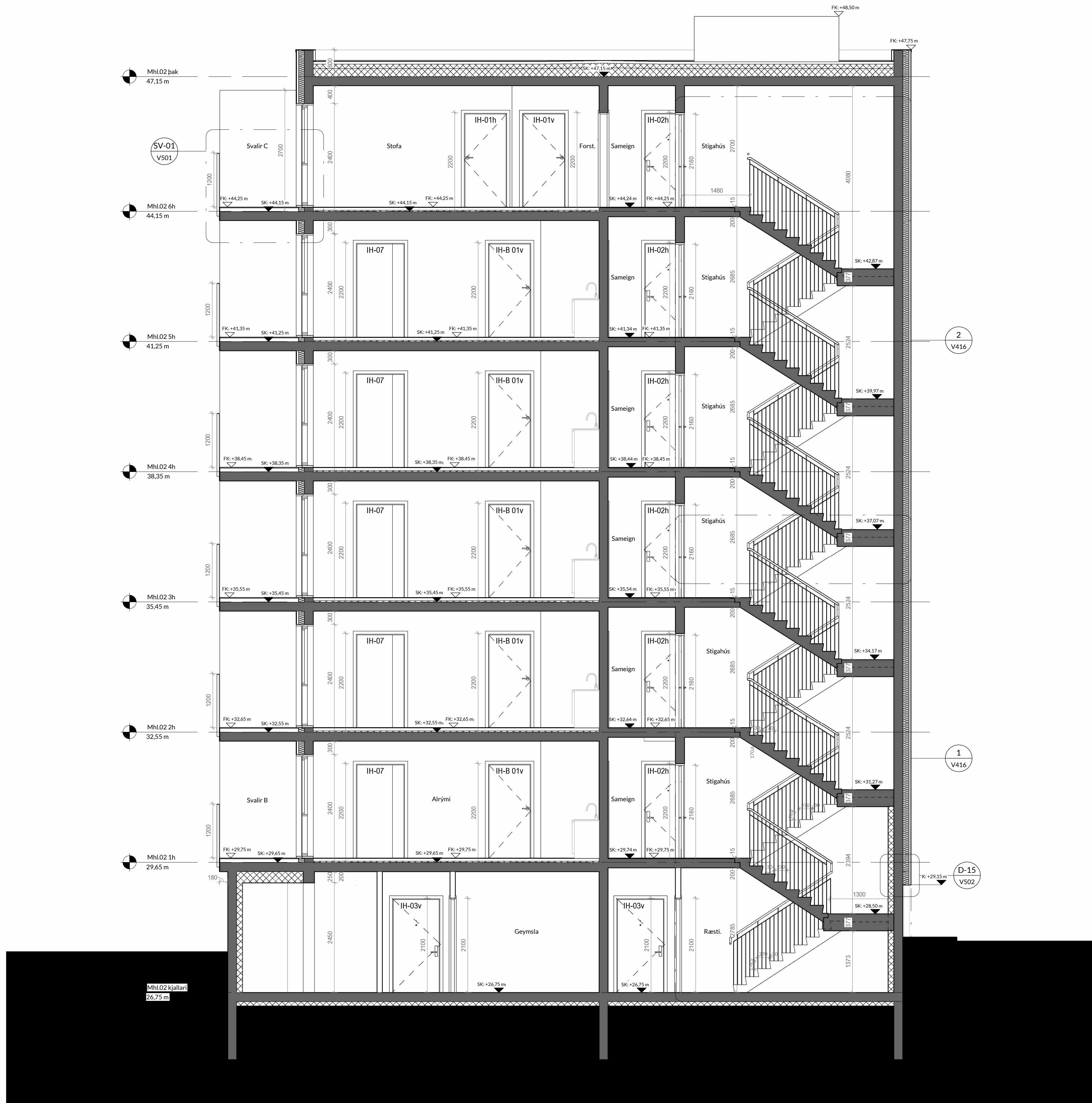
Skurðmynd 02 Mhl.01. 1:50
