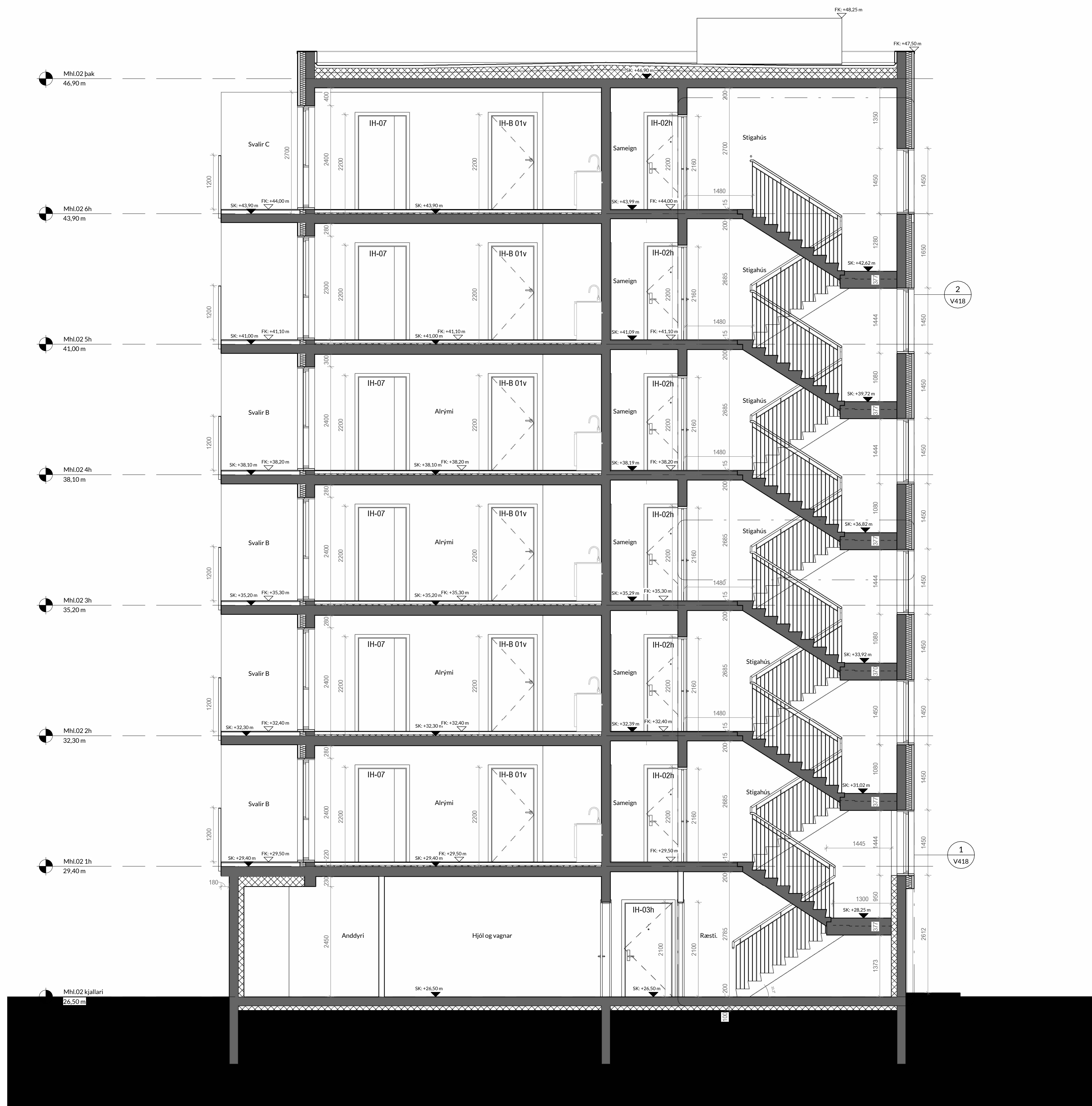
Skurðmynd 04 Mhl.02. 1:50
