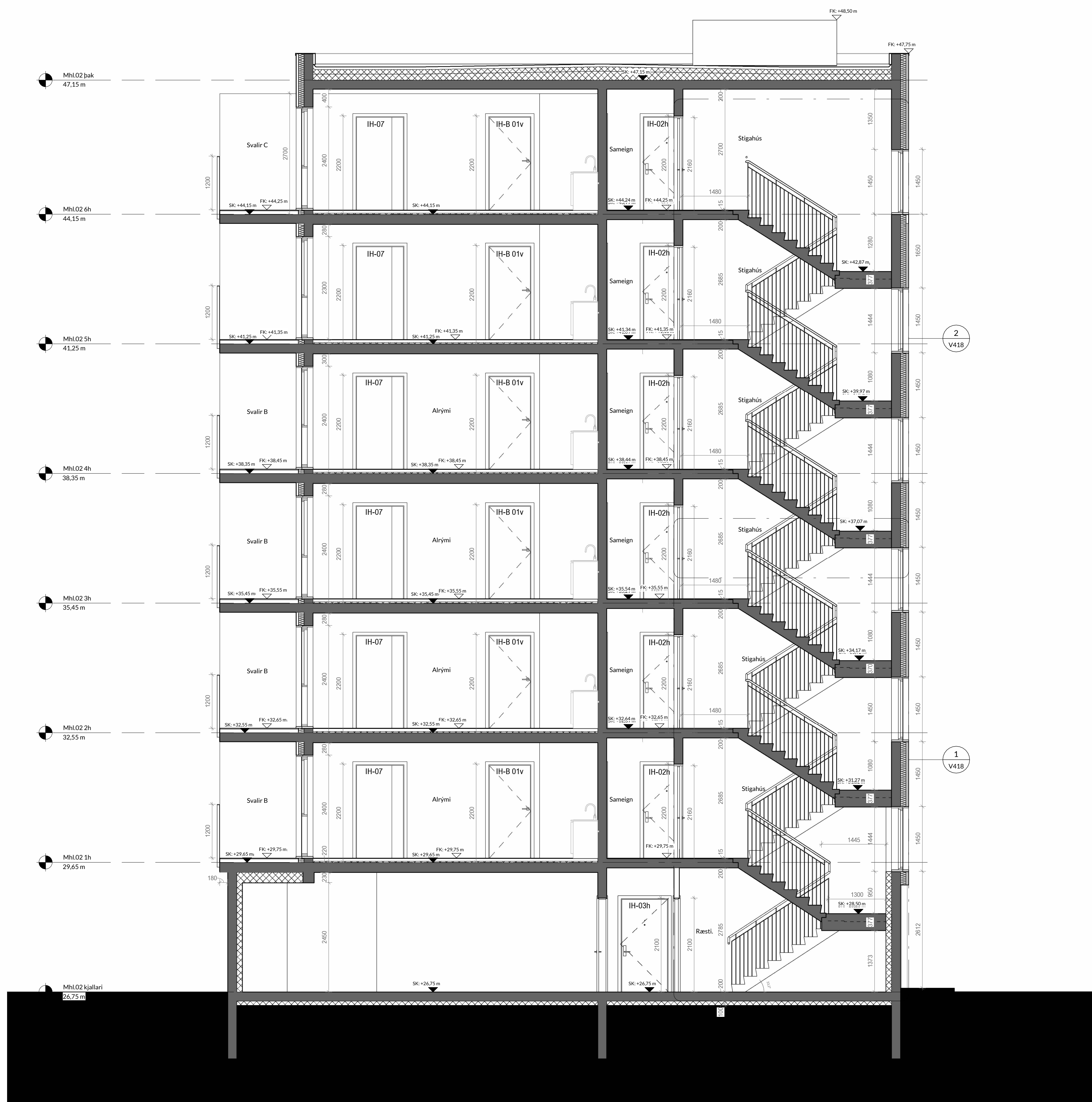
Skurðmynd 04 Mhl.01. 1:50
