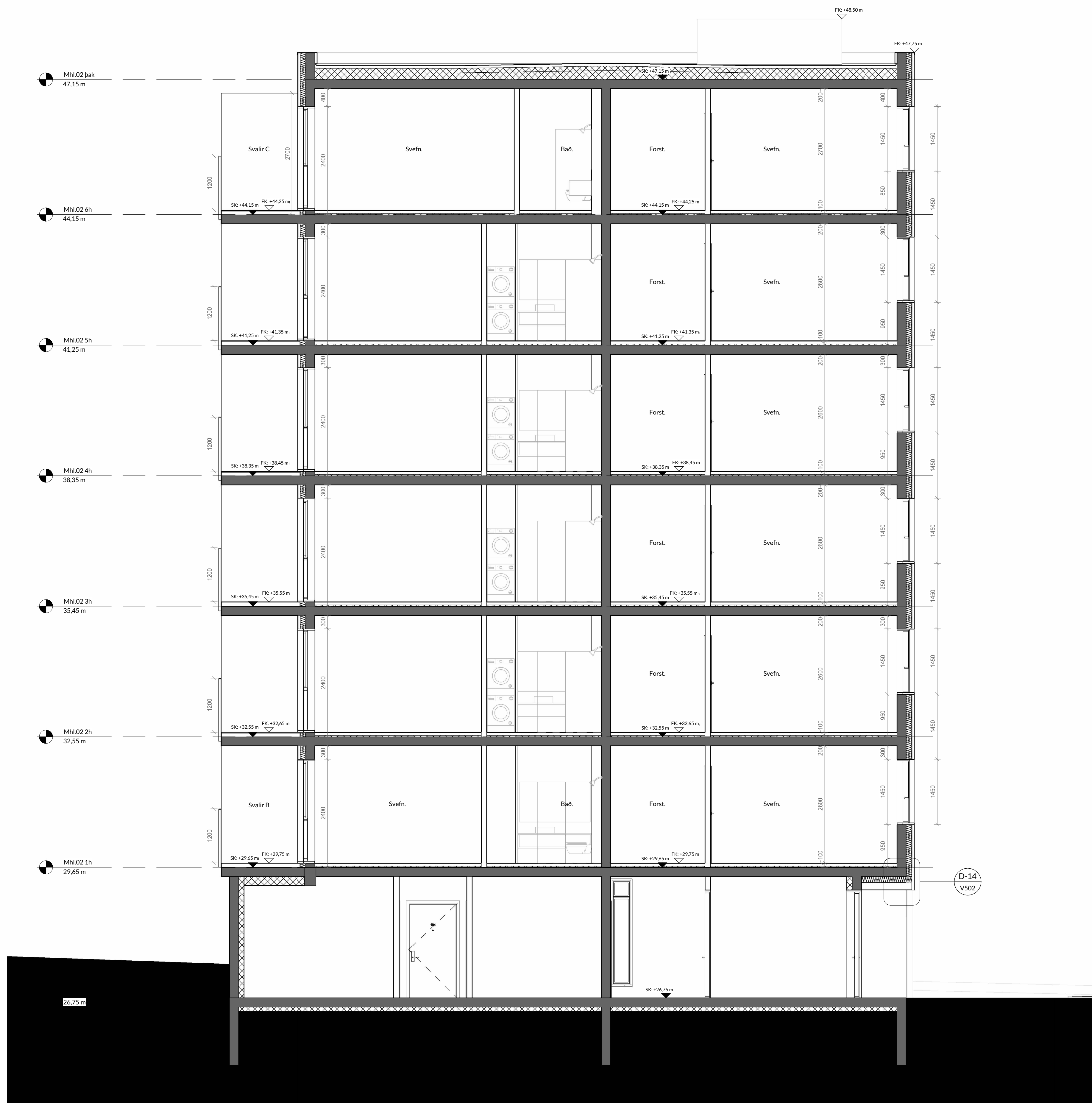
Skurðmynd 03 Mhl.01. 1:50
