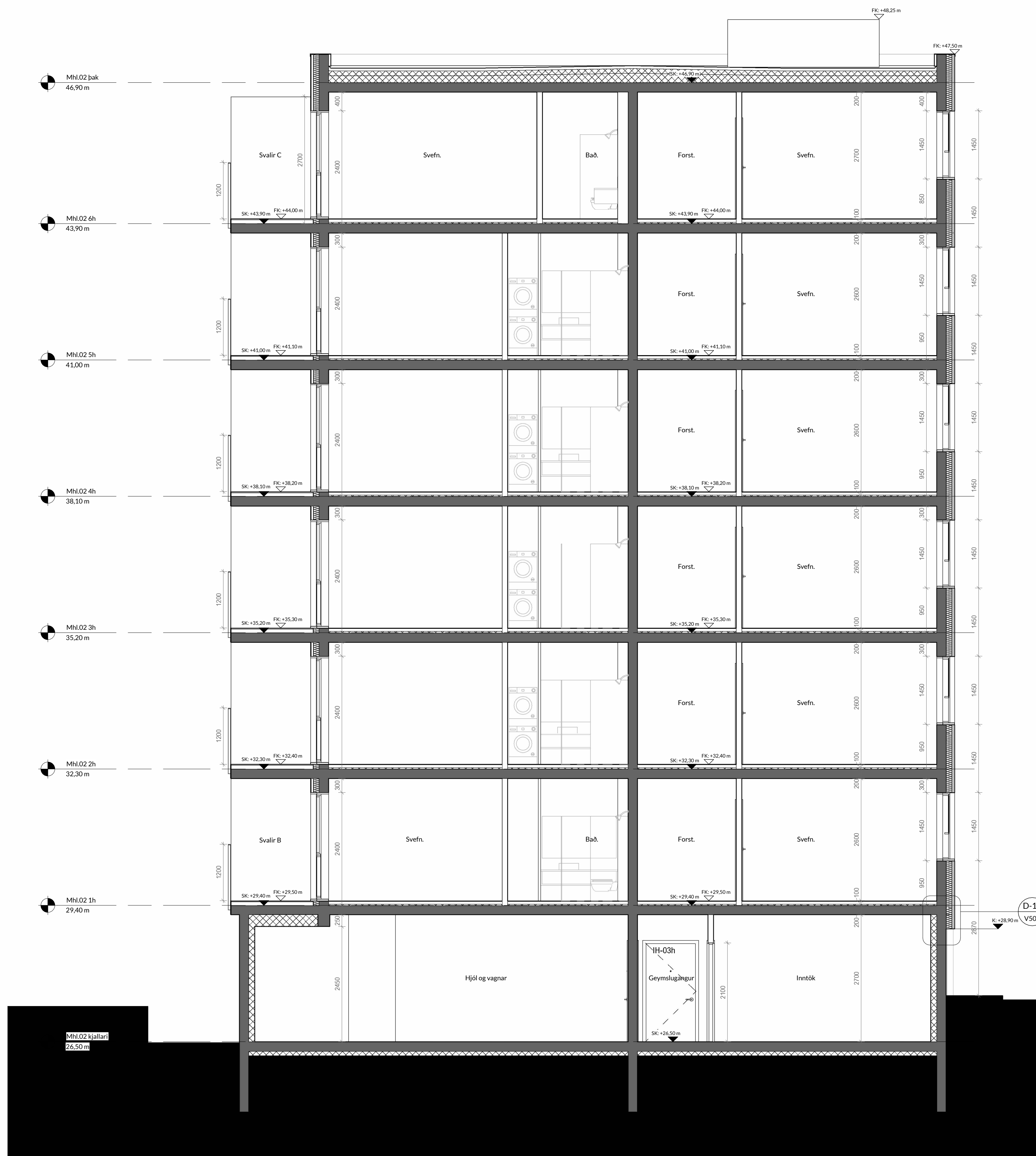
Skurðmynd 03 Mhl.02. 1:50
